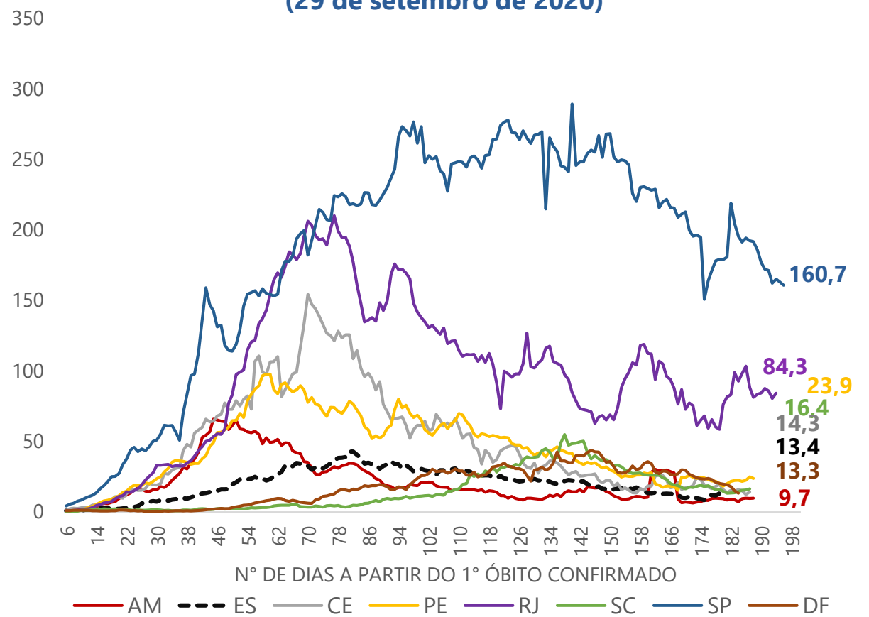
Evolução de novos óbitos diários - Média móvel de 7 dias (29 de setembro de 2020)
