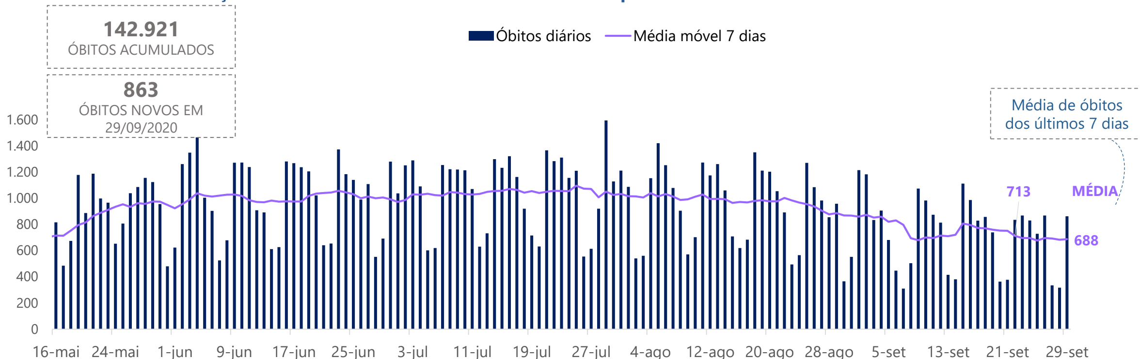
Evolução dos novos óbitos confirmados de Covid-19 por dia no Brasil e média móvel 7 dias
