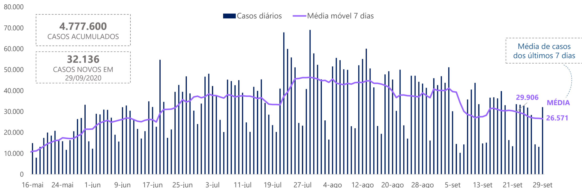
Evolução dos novos casos confirmados de Covid-19 por dia no Brasil e média móvel 7 dias
